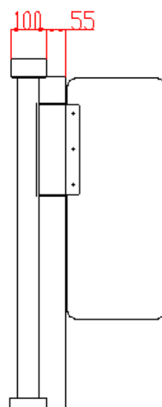
左视图
