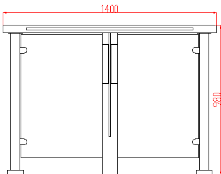
主视图
